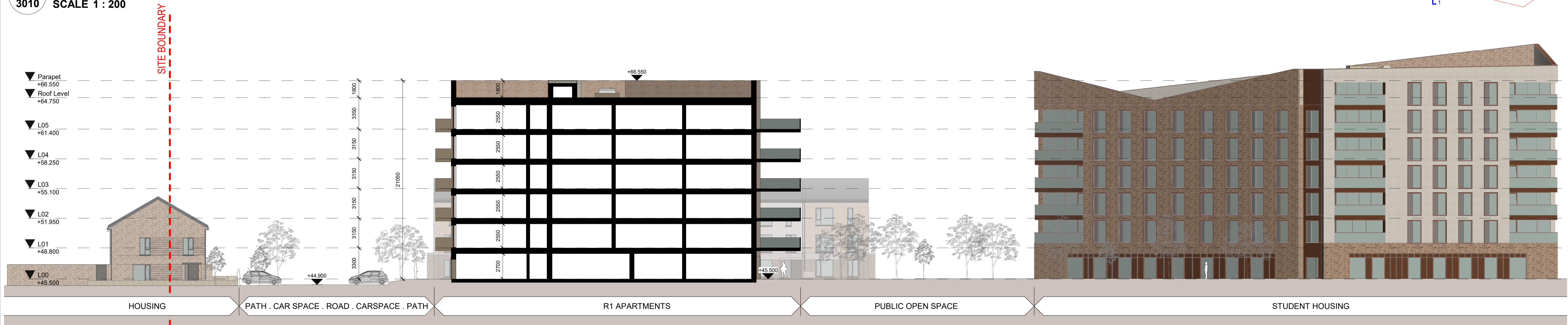
2 Section BB 3010 SCALE 1 : 200
