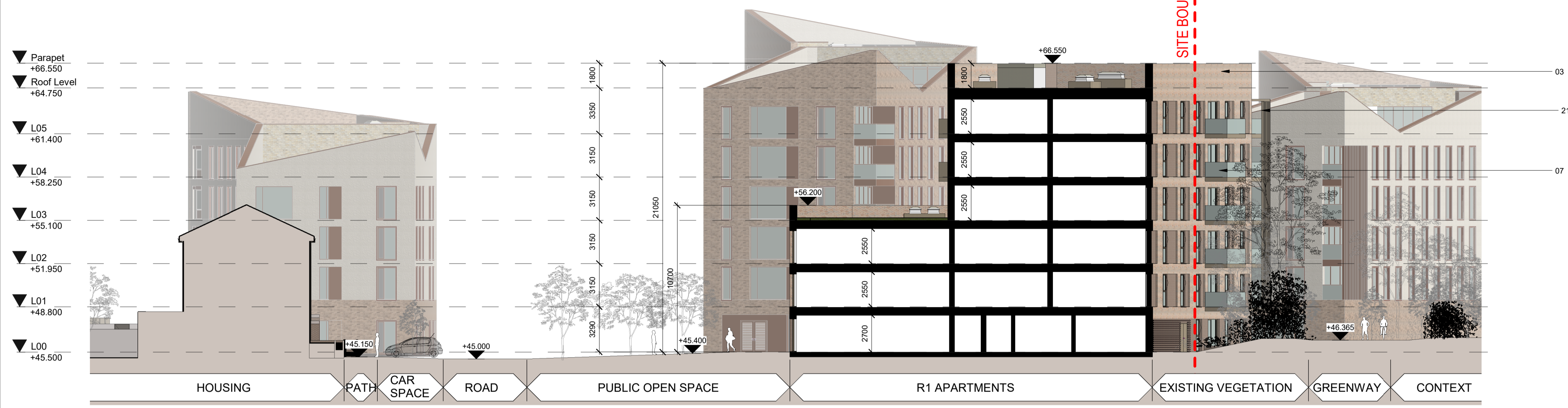
1 Section AA 3010 SCALE 1 : 200
